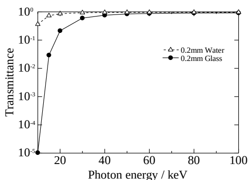
図4 2mm厚のガラス及び水に対する光子の透過率のエネルギー依存性。エネルギーが高いほど透過率は上昇するが、100keV 付近からそれほど大きく変化しないことが分かる。また低エネルギーでは物質による透過率の差が大きくなる。
