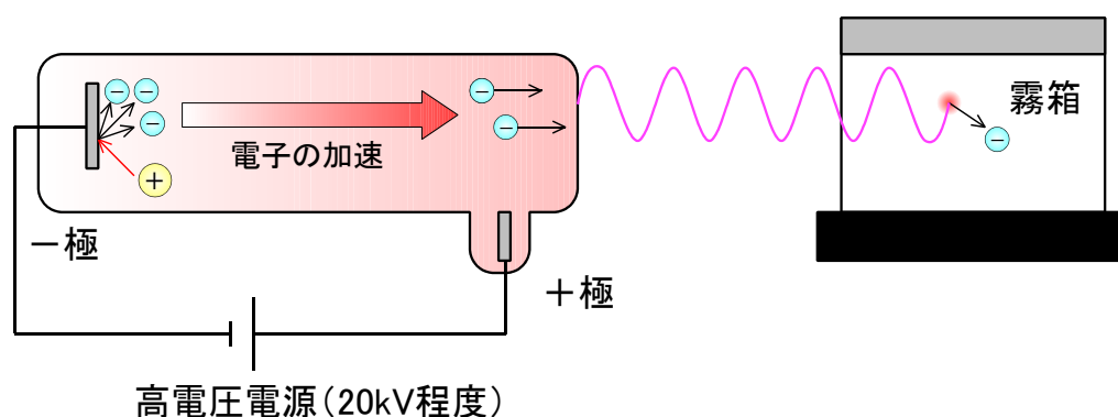
図 5 クルックス管の模式図と、電子から X 線、再び光電子に変化する様子。冷陰極において陽イオンが加速されて二次電子を叩き出し、陰極付近の電界によって加速されて電子ビームとなる。陰極ごく近傍以外では電界は弱く等速直線運動した後、ガラス管にぶつかり制動放射 X 線を放出し、電子は止まる (20 keV 程度では電子自体はガラス管を透過できない。特性 X 線も放出されるがエネルギーが低いとやはりガラス管を透過できない)。ガラス管を透過した制動放射 X 線は、2 \pi 方向に拡散していき、距離の二乗に従って強度が小さくなる。最終的に空気原子にぶつかり光電効果を起こし、光電子を叩き出す。霧箱を用いると、空気中での飛程 5 mm 程度のこの光電子を観察することが出来る。
