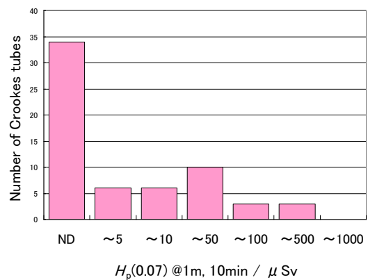
図2 2018年度に実施した暫定ガイドライン設定以前の実態調査結果。NDは検出限界(50 \mu\text{Sv}@20\text{ cm} )以下。
