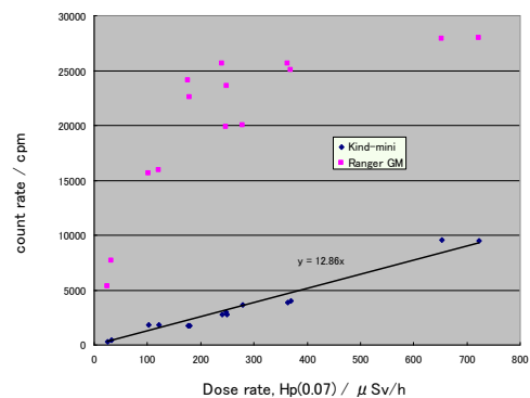
図 7 プラスチックシンチレーターを用いた簡易型サーベイメーター Kind-mini とパンケーキ型 GM サーベイメーター Ranger を用いた線量率と計数率の相関。線量率は電離箱を用いて測定した。
