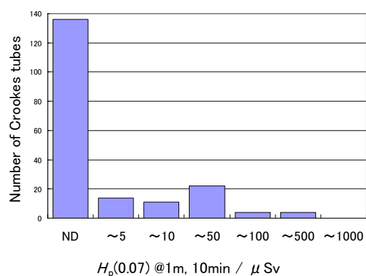
図3 2019年度に実施した暫定ガイドライン準拠(放電極距離20 mm)での実態調査結果。NDは検出限界(50 \mu\text{Sv}@20\text{ cm} )以下。
